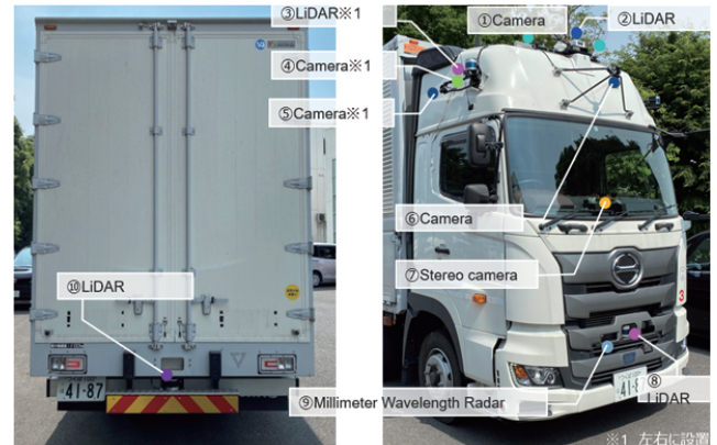
図4 各種センサを搭載した実証実験用トラック
