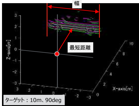
点群比較
