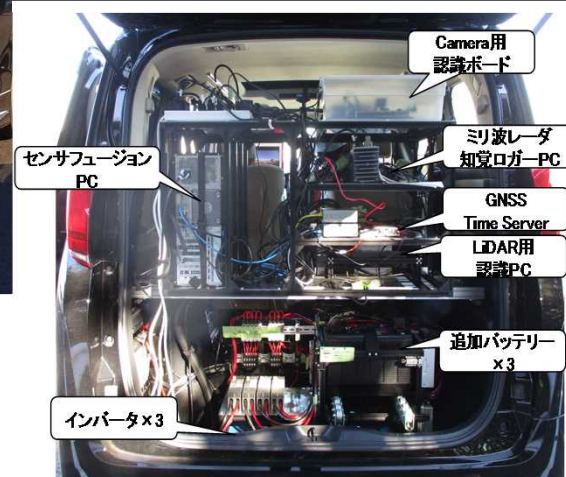
車室内架台
